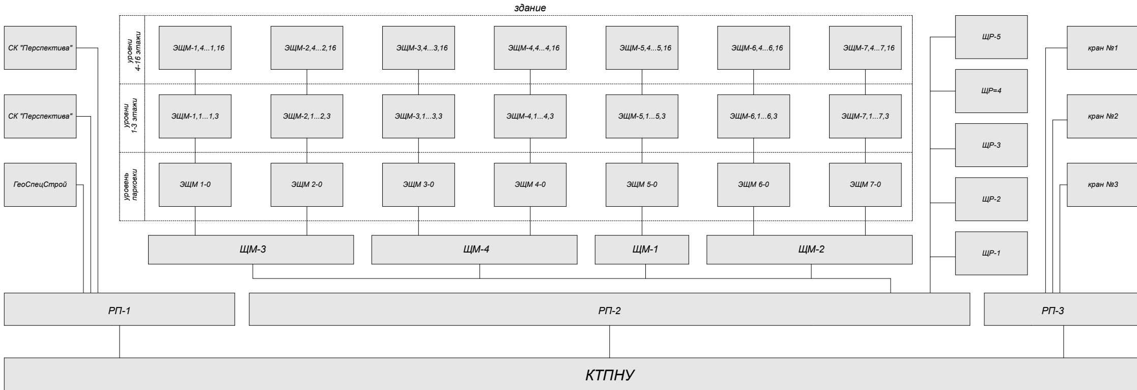
Схема структурная электропитания строителиной площадки по адресу: Москва, улица Автозаводская, дом 24, кор.1
