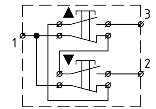
Принципиальная схема SBn
