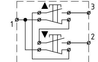
Принципиальная схема SBn
